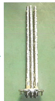
スケールが付着し、交換が必要となったヒーター
